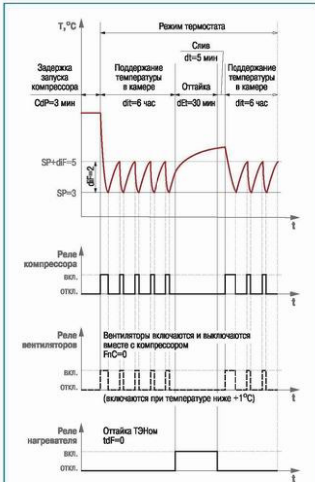
▲ Пример работы TRM974 в режиме ТЕРМОСТАТ: график изменения температуры в камере и временные диаграммы работы выходных реле (для значений параметров, установленных по умолчанию на заводе-изготовителе)
