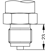
G 1/2" EN 837 M 20x1,5
