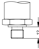
G 1/4" DIN 3852 M 10x1 M 12x1,5
